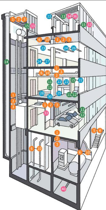
RC/S造
